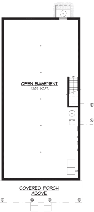
BASEMENT PLAN SCALE: N.T.S. 1,334 SQFT. GROSS AREA
